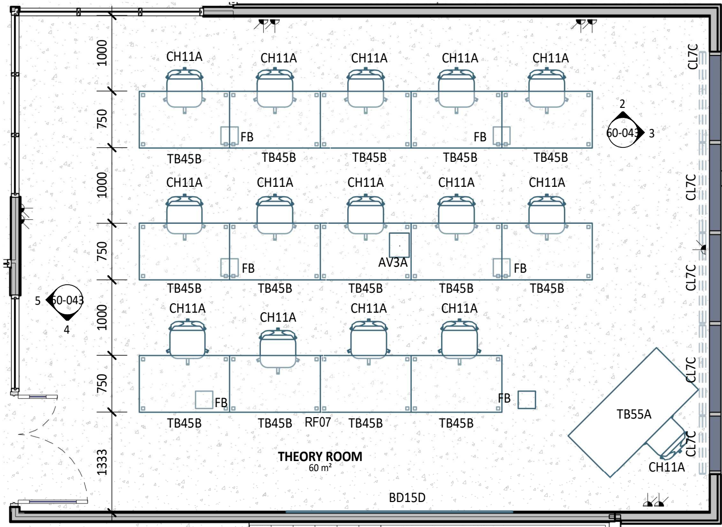
1 PLAN DETAIL 1 : 50
